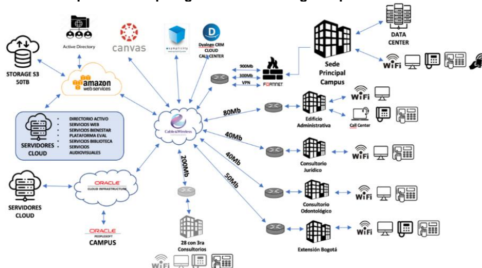
Ilustración N°5. Arquitectura topológica de la tecnología implementada en la Universidad.
